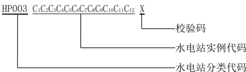
图 11 水电站代码结构
