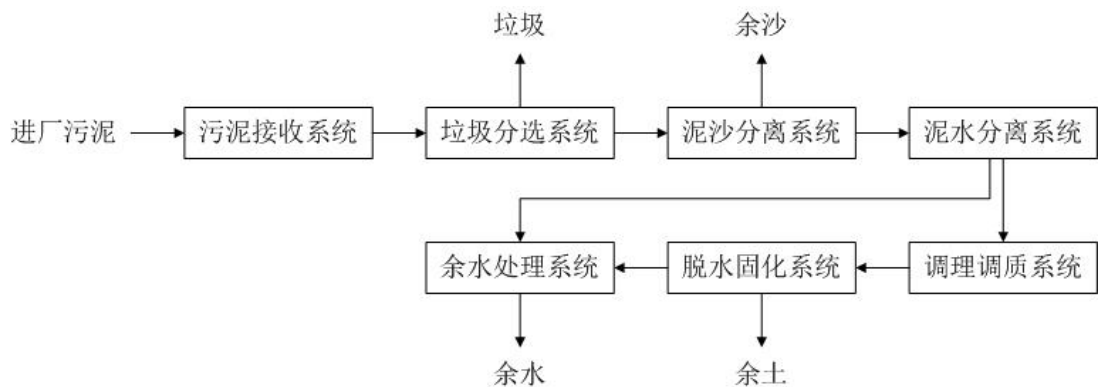
图 1 污泥处理工艺流程
